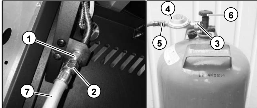
Abb. 1 - Gas anschließen
