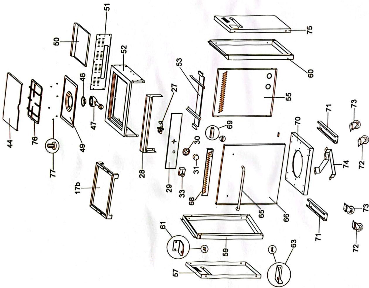
Sprengezeichnung Eden 100
